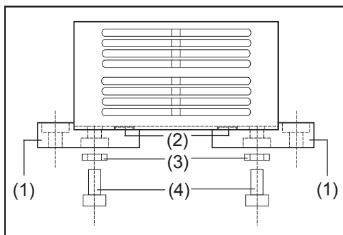
Afb. 3 Optie vloermontage
